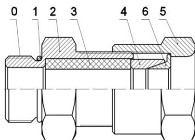
KBБ – для монтажа бронированного кабеля
