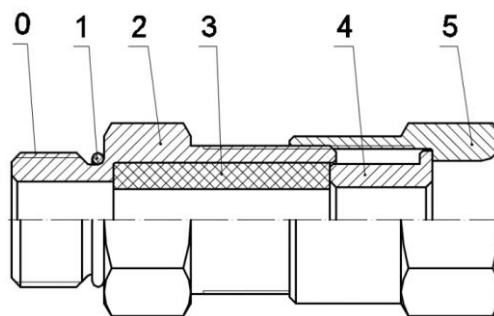
KBН – для монтажа открытого кабеля
