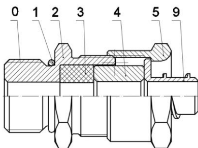
KBМ – для монтажа кабеля в металлорукаве
