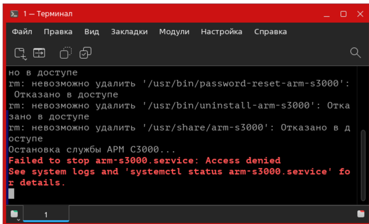
Рисунок 20. Ошибка доступа при удалении APM «C3000»
